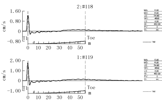
图 3 71 号桩加固后低应变检测波形
