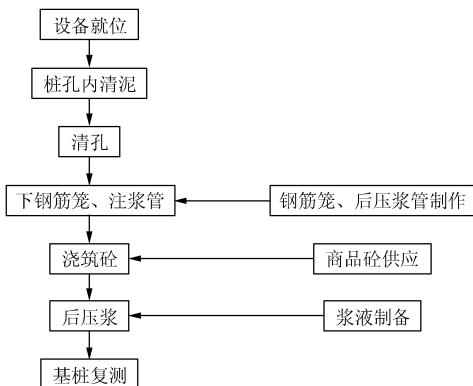
图1 施工工艺流程图
