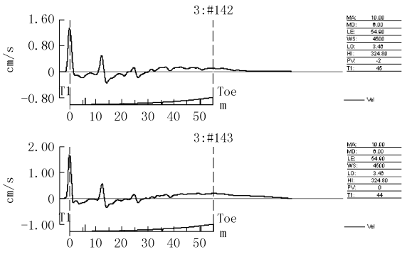
图 2 71 号桩加固前低应变检测波形
