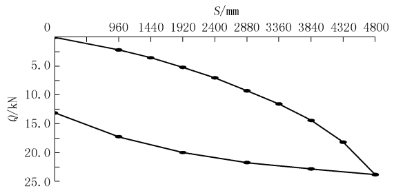
图 5 71 号桩静载试验 Q~s 实测曲线图
