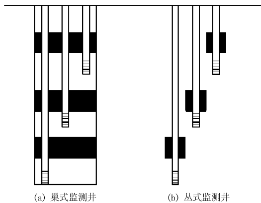
图 1 巢式监测井和丛式监测井示意图
