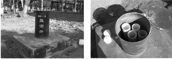
图2 安装好的巢式监测井
