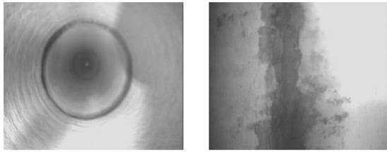
(a) 行走时拍摄的管道内壁图像 (b) 摄像头转动90°拍到的接缝图像
