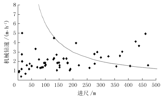
图4 三开营城组地层钻头综合评价结果图
