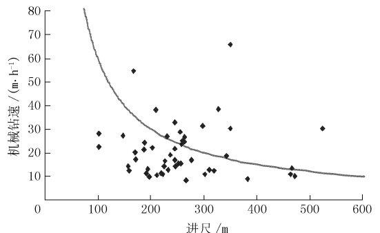
图 2 一开钻头综合评价结果图
