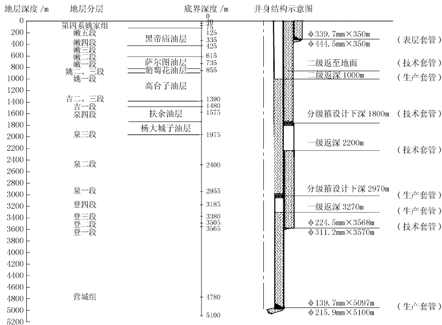
图 1 莺深 2 井井身结构设计
