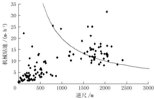
图3 二开 PDC 钻头综合评价结果图
