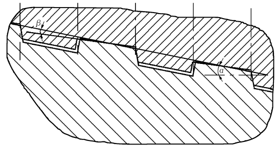
图1 梯形螺纹新结构
