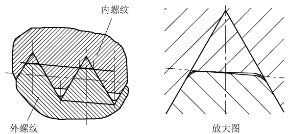
图2 API螺纹新结构
