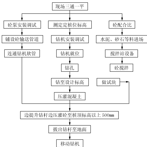
图 1 素混凝土桩施工工艺流程图
