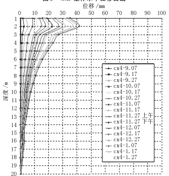
图6 CX4 土体水平位移曲线
