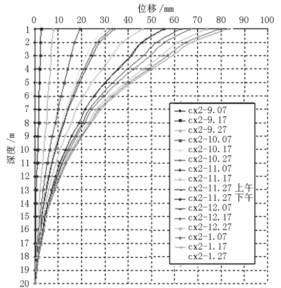
图4 CX2 土体水平位移曲线
