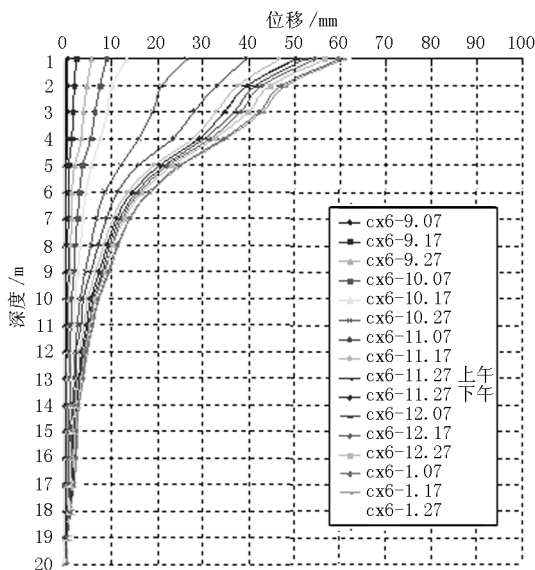
图8 CX6 土体水平位移曲线
