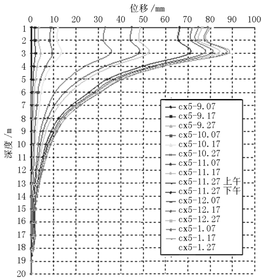
图7 CX5 土体水平位移曲线
