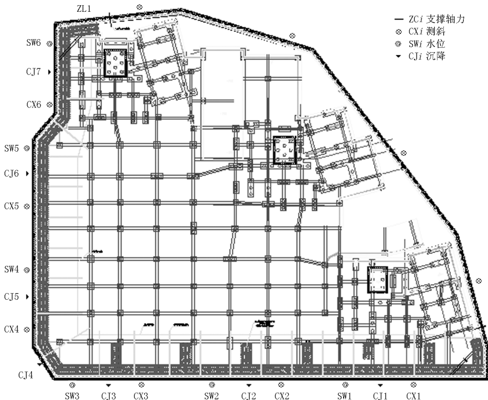
图 2 基坑监测平面布置图
