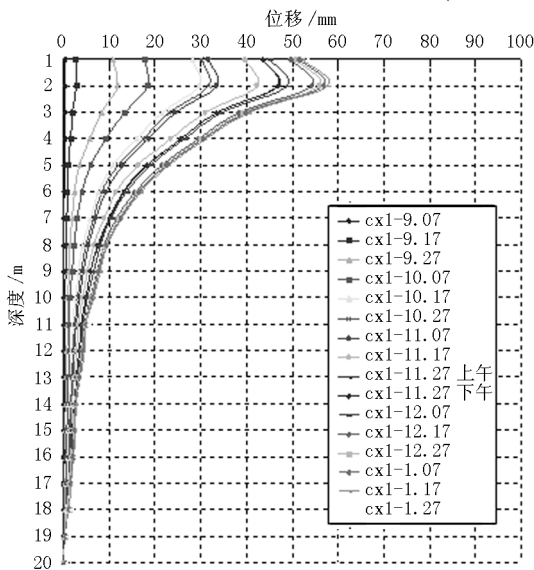
图3 CX1 土体水平位移曲线
