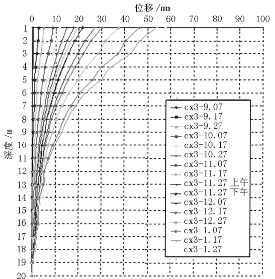
图5 CX3 土体水平位移曲线
