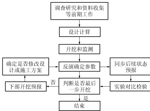
图 1 基坑开挖动态预报示意图
