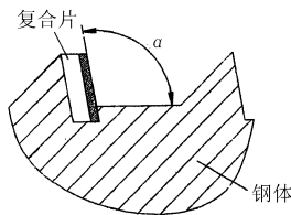
图 3 切削角 \alpha 示意图
