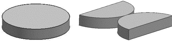
图5 复合片切削块保径示意图
