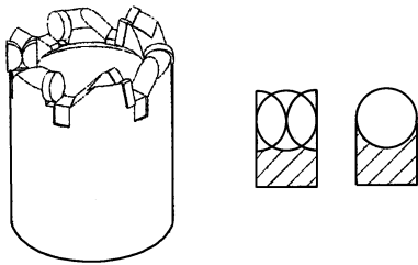
图 1 复合片的排列
