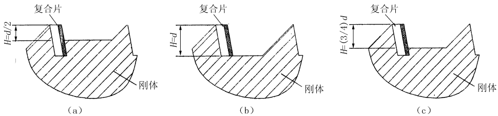
图 2 复合片出露刚体高度 H 与复合片直径 d 的关系示意图
