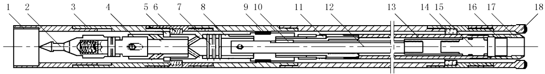
图 1 液压剪切式取样钻具结构
