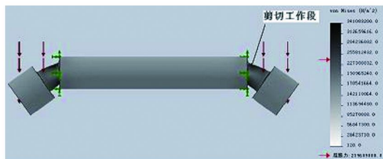
图 2 剪切销应力状态及变形
