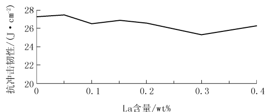
图2 稀土 La 对胎体抗冲击韧性的影响
