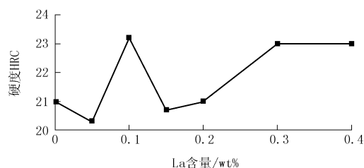
图3 稀土 La 对胎体硬度的影响
