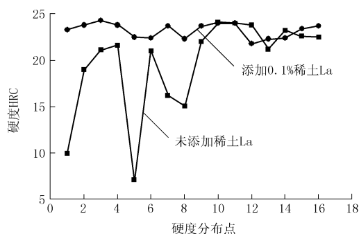
图4 稀土添加前后硬度测量统计图
