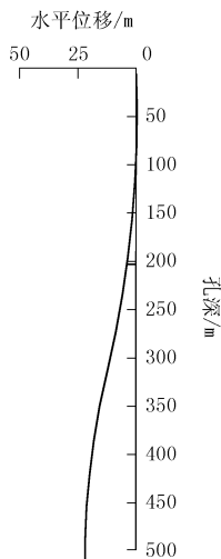
图4 钻孔纠斜轨迹图
