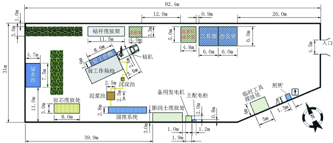
图 4 钻场布置图
