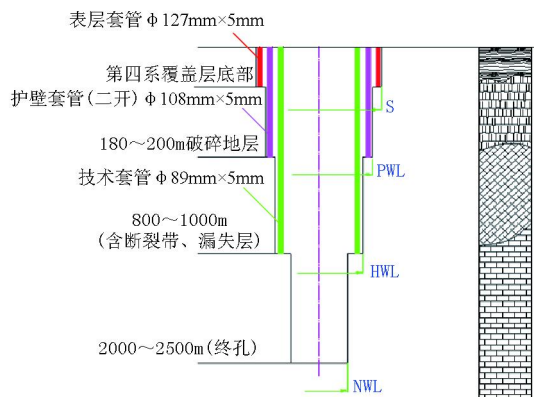
图2 钻孔结构示意图
