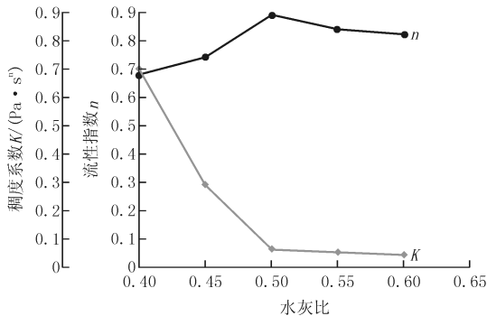
图1 不同水灰比影响下的水泥流变特性规律
