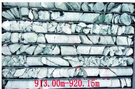
图3 破碎段岩心
