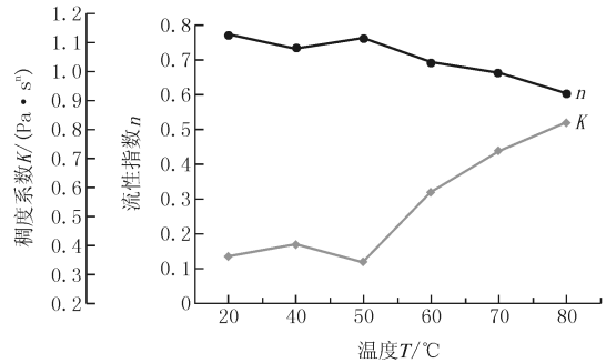
图2 不同温度影响下的水泥浆流变特性规律
