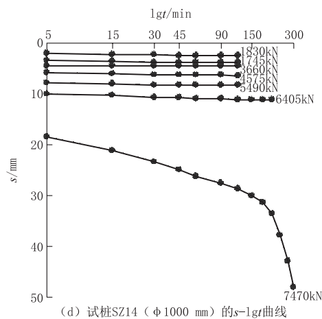
图 2 未注浆试桩典型 Q-s 和 s-lgt 曲线
