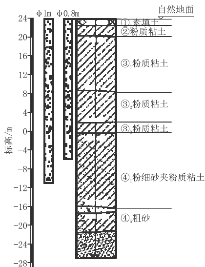
图 1 试桩地层剖面
