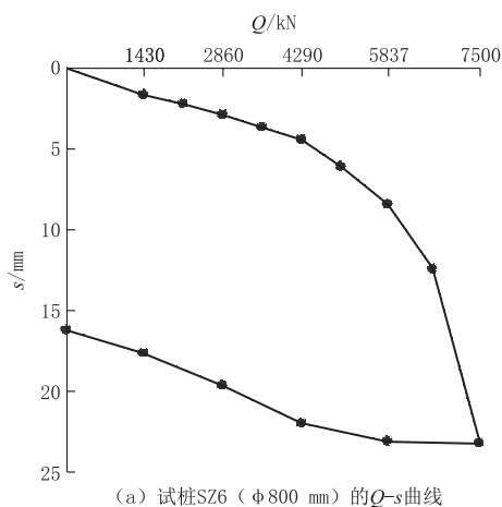
(a) 试桩SZ6 (φ800 mm) 的Q-s曲线
