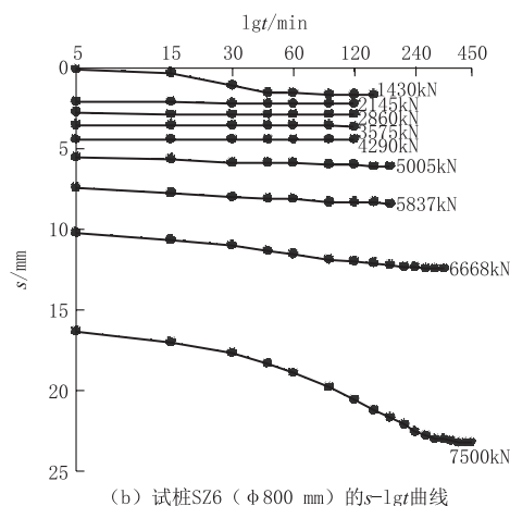
(b) 试桩SZ6 (φ800 mm) 的s-lgt曲线
