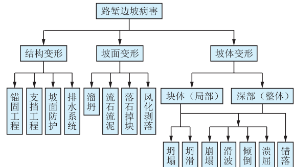
图6 公路边坡工程病害分类图
