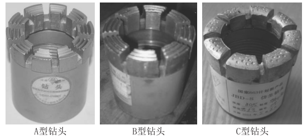
图 2 实验钻头
