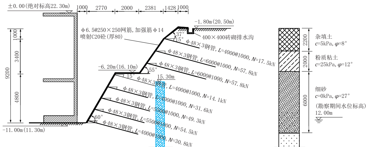
图2 基坑西侧土钉墙剖面
