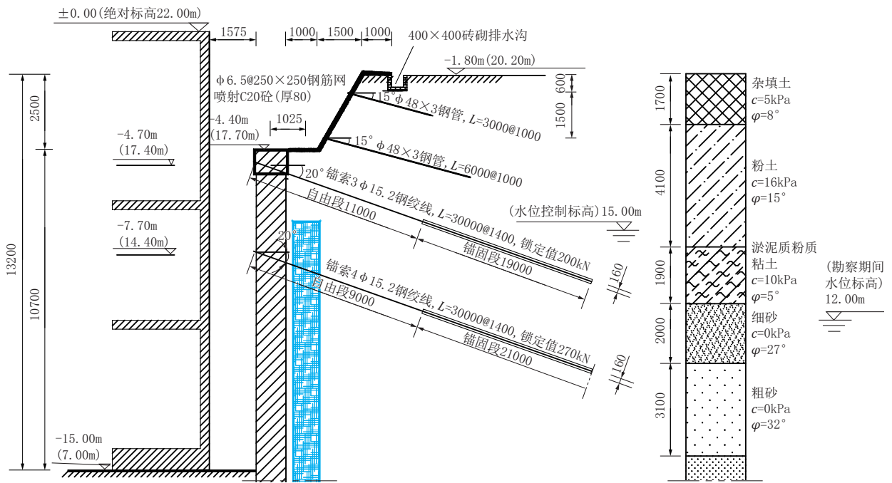
图4 基坑东侧土钉墙+桩锚支护剖面
