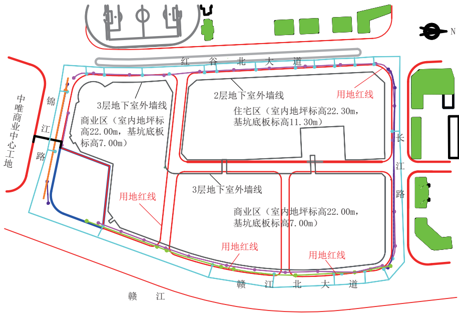
图1 基坑周边环境
