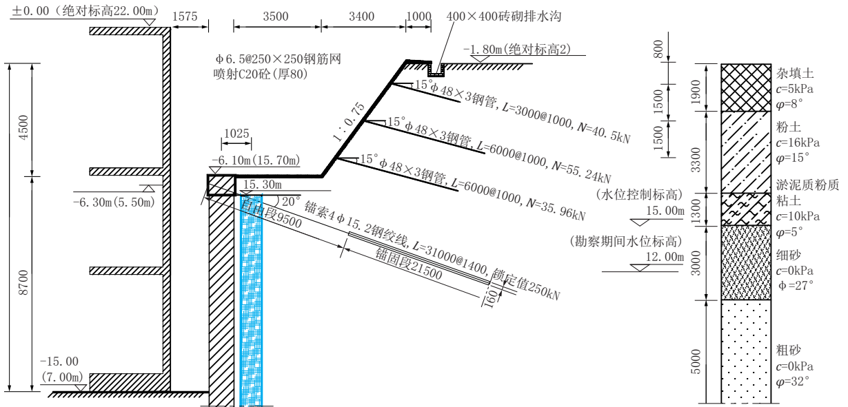
图 3 基坑北侧土钉墙+桩锚支护剖面
