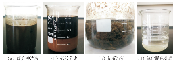
图6 废弃冲洗液处理工艺
