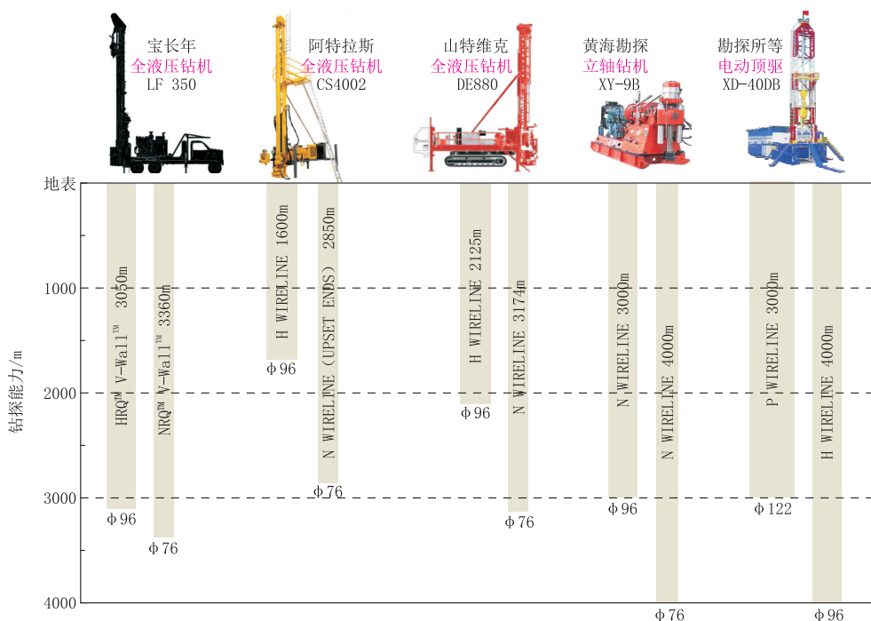
图 1 各国地质钻探装备钻深对比
