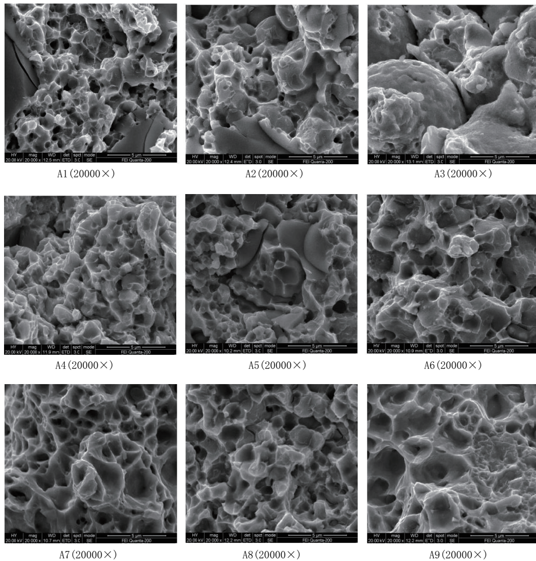
图7 断口截面SEM图像
