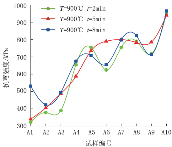
图4 不同配方的抗弯强度变化(空白试样)
