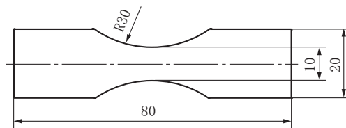
图1 拉伸试样的尺寸
