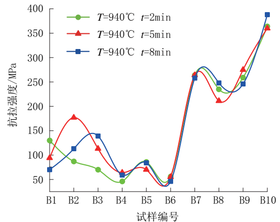
图3 不同配方的抗拉强度变化(加金刚石试样)
