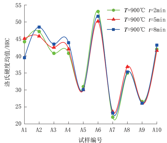
图6 不同配方的硬度变化(空白试样)
