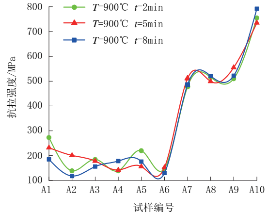
图2 不同配方的抗拉强度变化(空白试样)
