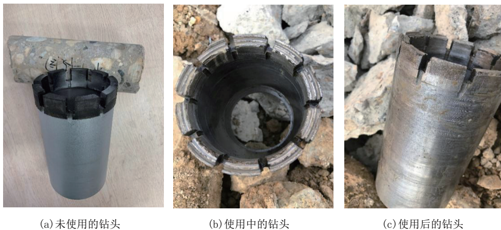
图8 现场使用的金刚石钻头
