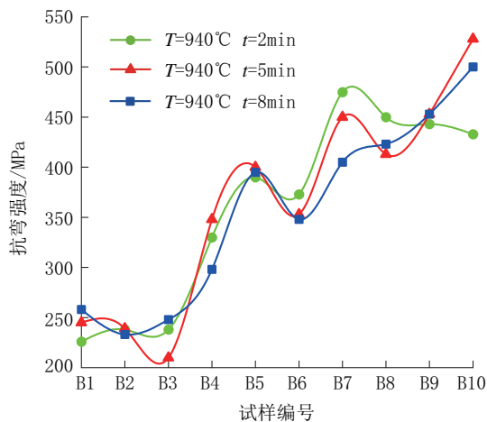
图5 不同配方的抗弯强度变化(加金刚石试样)
