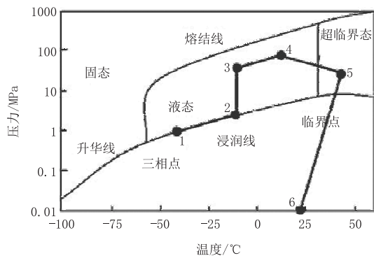
图1 二氧化碳相图
