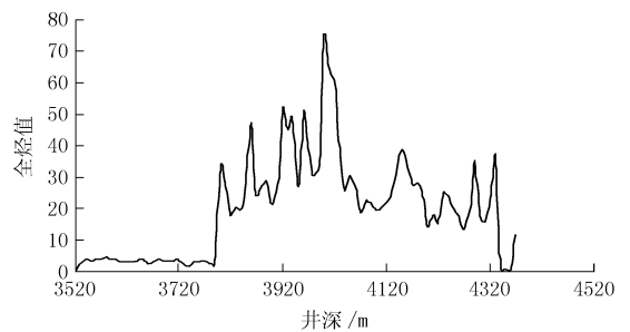
图 1 四开欠平衡段全烃值曲线图
