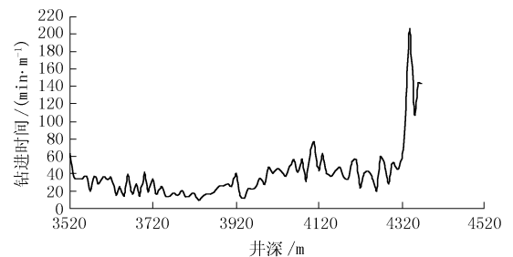
图 2 四开欠平衡段钻时曲线图
