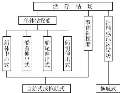
图1 主要漂浮钻场分类
