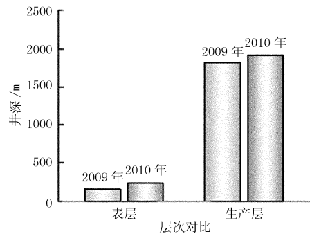
图 1 2009、2010 年中浅层探井井身结构对比
