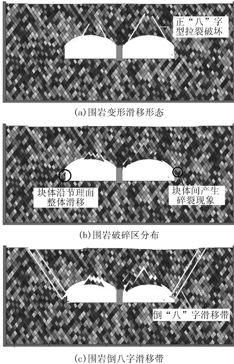
图2 K22+402断面围岩变形破坏过程
