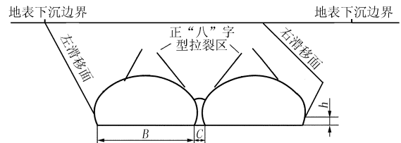
图5 深埋隧道围岩破坏区域分布图
