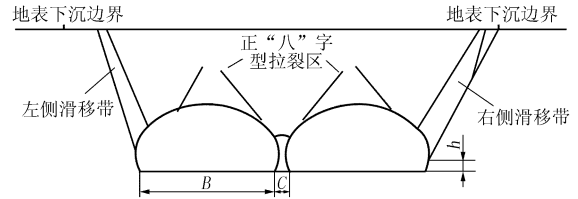
图4 浅埋隧道围岩破坏区域分布图
