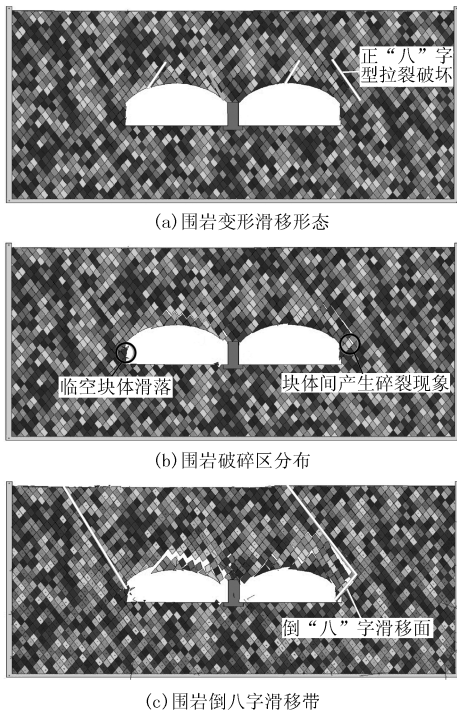
图3 K22+562断面围岩变形破坏过程
