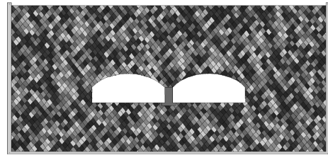
图 1 金鸡山隧道计算模型
