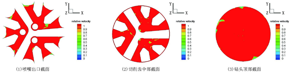
图 8 流场不同截面速度分布
