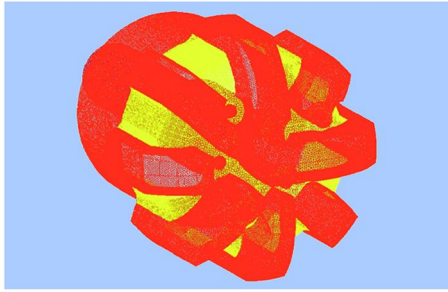
图5 低温电铸孕镶脉冲石油钻头网格示意图
