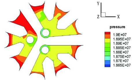
图6 喷嘴出口截面压力分布(Pa)
