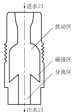
图 11 脉冲喷嘴示意图
