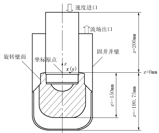
图4 计算区域示意图
