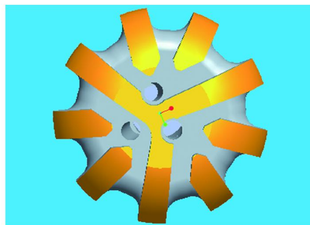
图 1 低温电铸孕镶脉冲石油钻头三维图
