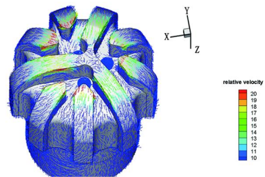
图 9 钻头表面相对速度矢量图
