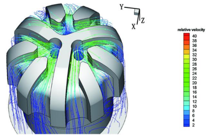
图7 计算区域相对速度的流线分布
