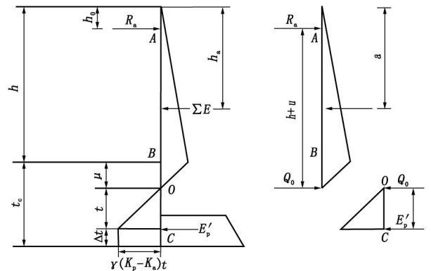
图 8 简化等值梁法计算原理
