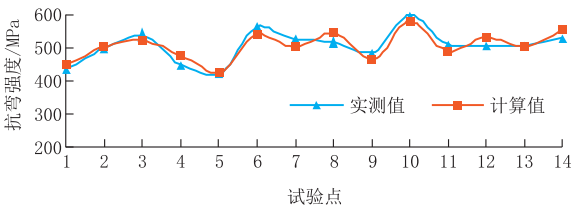
图 2 含金刚石胎体抗弯强度回归方程拟合效果
