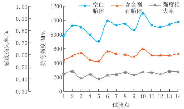
图 3 试样的抗弯强度与强度损失率
