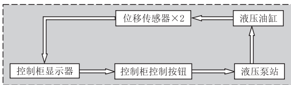
图5 监测控制系统
