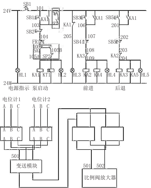
图6 电控监测系统原理
