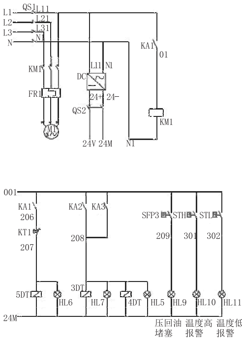
图6 电控监测系统原理
