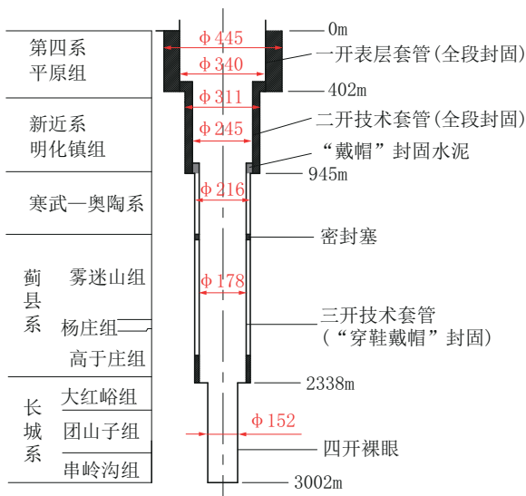
图 4 JK01 地热井成井结构示意图
