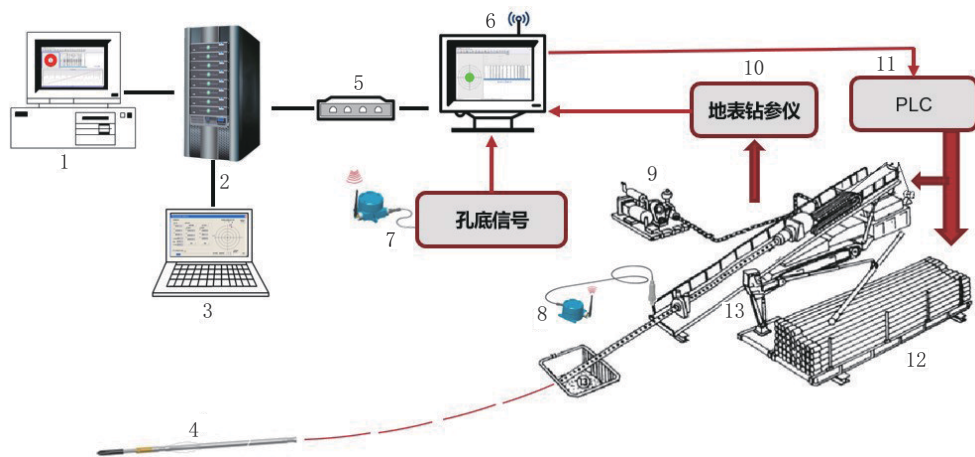
1—数据中心;2—服务器;3—远程监视器;4—孔底组合钻具;5—交换机;6—近机工控显示系统;7、8—传感器;9—泥浆泵;10—地表钻参仪;11—PLC;12—钻杆;13—定向钻机
